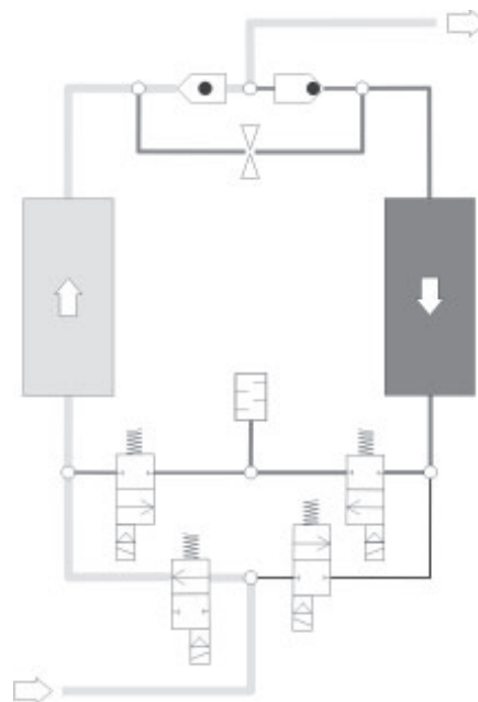
Fáze opětovného tlakování
